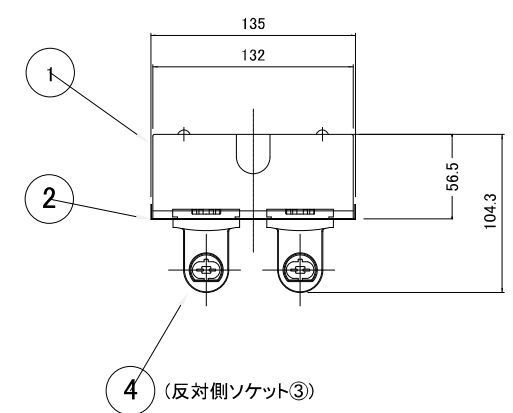
背面図
